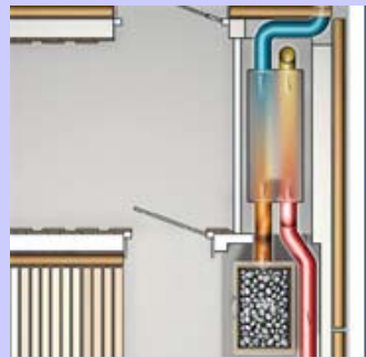
Bild: Beispiel einer Sauna internen Wärmerückgewinnung (Quelle Klafs)
